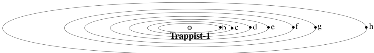
מערכת TRAPPIST-1
