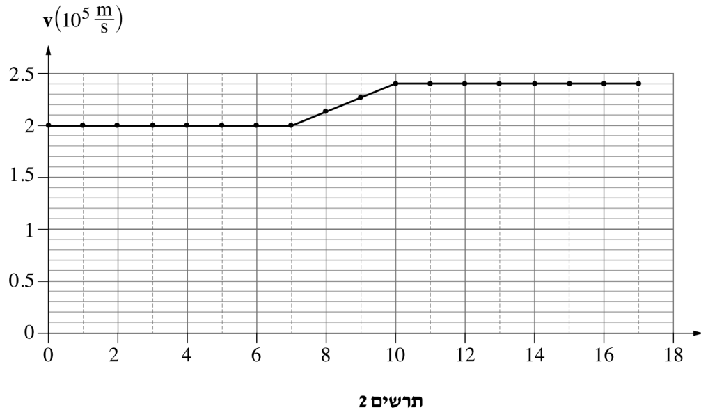
גודל מהירות הפרוטון כפונקציה של הזמן
