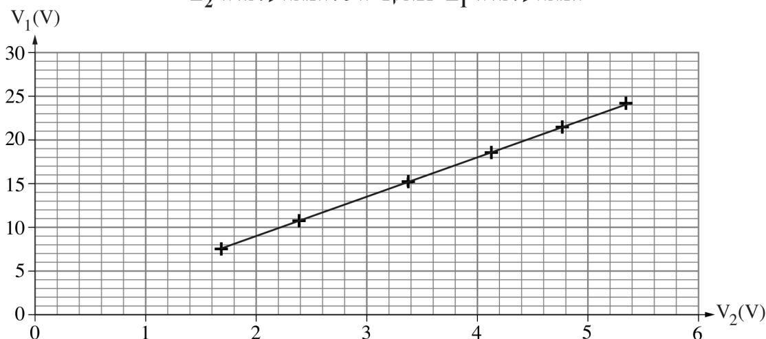
המתח על נורה L_1 כפונקציה של המתח על נורה L_2
